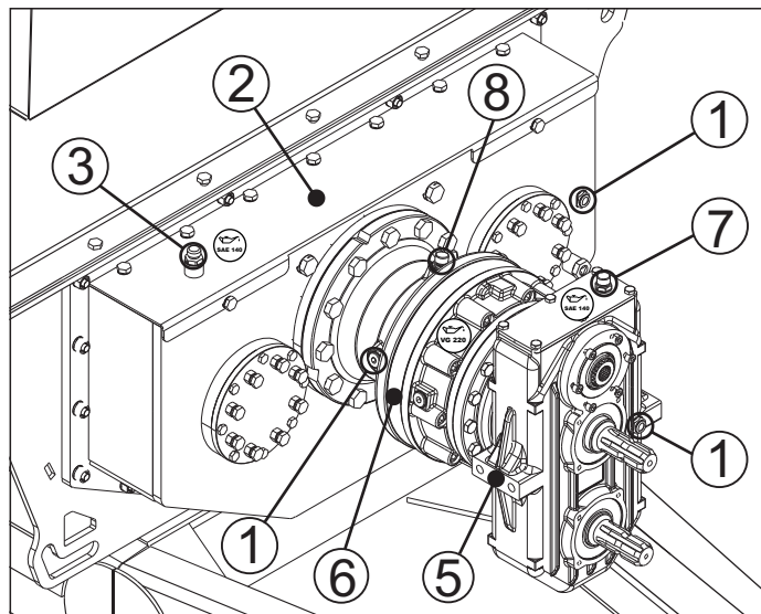
Fig. 22 - Caixa de Engrenagen e Planetário
